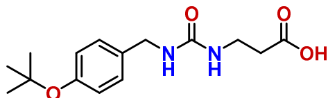
3-(3-(4-(Tert-butoxy)benzyl)ureido)propanoic acid
